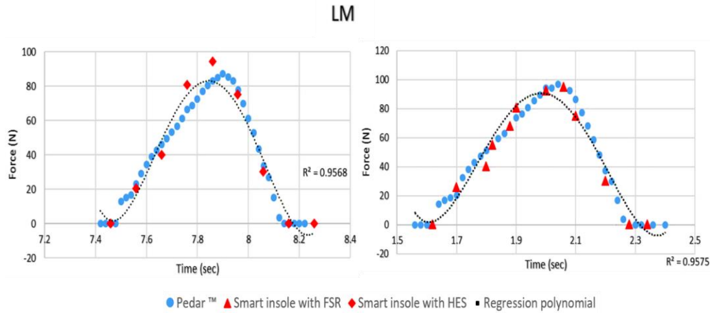
شکل ۱۱- نتایج همبستگی و تطبیق LM دو نمودار حاصل از پدار و کفی اثر هال و کفی FSR با ضریب رگرسیون ۰/۹۶ و ۰/۹۶
