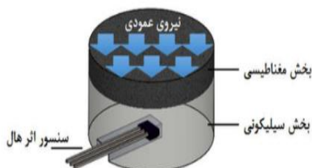
شکل ۲- نمایش شماتیک بخش‌های مختلف سنسور
