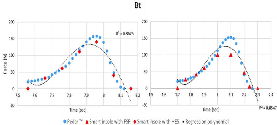
شکل ۱۵- نتایج همبستگی و تطبیق Bt دو نمودار حاصل از پدار و کفی اثر هال و کفی FSR با ضریب رگرسیون ۰/۸۷ و ۰/۸۵
