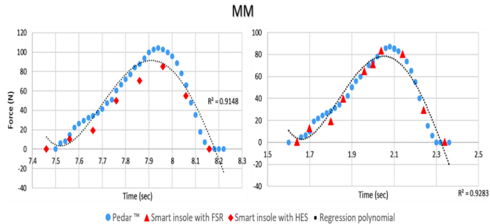
شکل ۱۳- نتایج همبستگی و تطبیق MM دو نمودار حاصل از پدار و کفی اثر هال و کفی FSR با ضریب رگرسیون ۰/۹۱ و ۰/۹۳
